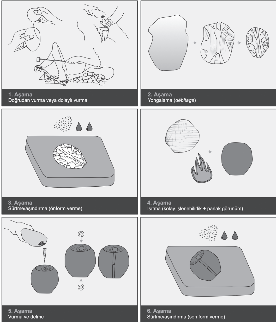
Figür 2: Kalsedon grubu sert ve yongalanabilir taşlardan üretilmiş kelebek formlu boncuklar için önerilen üretim zinciri (Çizimde Alarashi 2014, Figür 15.3; Inizan, Reduron-Ballinger, Roche ve Tixier, 1999, Figür 4; Roux, Brill ve Dietrich, 1995, Figür 1'den yararlanılmıştır).
